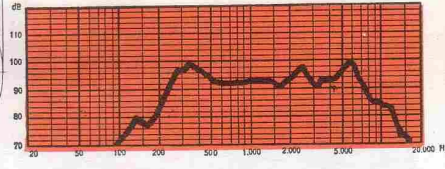
CIS 12 D 127 mm - 5" 2 W
