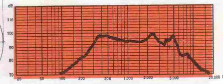
CIS 8 C 77 mm - 3" 0,4 W
