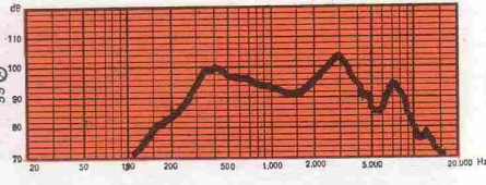
CIS 9 C 92 mm - 3 5/8" 0,6 W
