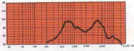
CIS 7 B 70 mm - 2 25/32" 0,3 W
