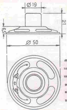
CIS 5 B 50 mm - 5" 0,15 W
