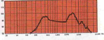
CIS 7 C 66 mm - 2 9/32" 0,3 W
