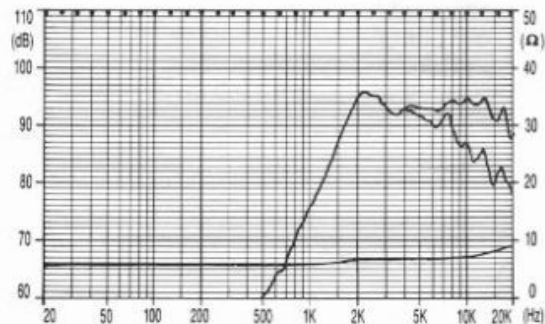
Courbe de réponse dans l'axe et à 30° hors de l'axe Courbe d'impédance
