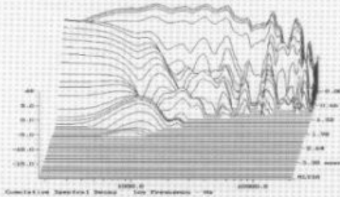
Zerfallsspektrum / Waterfall
