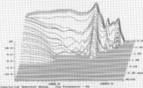
Zerfallsspektrum / Waterfall
