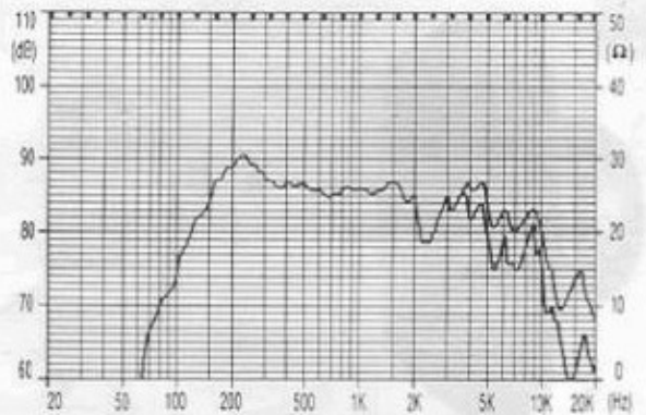
Courbe de réponse dans l'axe et à 30° hors de l'axe
